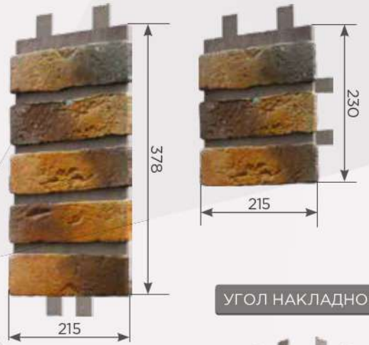
ОБРАМЛЕНИЕ ВЫСОТОЙ 3 И 5 КИРПИЧА
