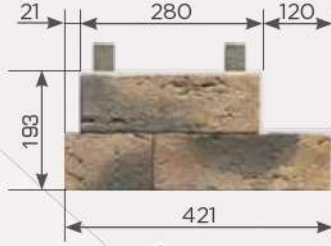
УГОЛ СОСТАВНОЙ ПРАВОЙ
