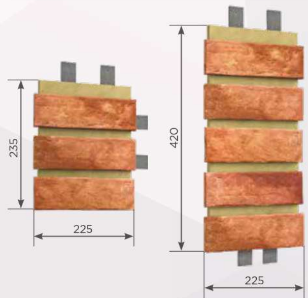
ОБРАМЛЕНИЕ ВЫСОТОЙ 3 И 5 КИРПИЧА
