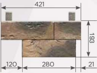
УГОЛ СОСТАВНОЙ ЛЕВЫЙ
