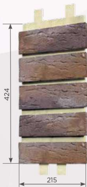
ОБРАМЛЕНИЕ ВЫСОТОЙ 3 И 5 КИРПИЧА
