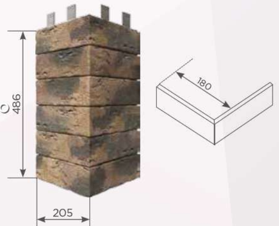
УГОЛ В ПЛОСКОСТИ
