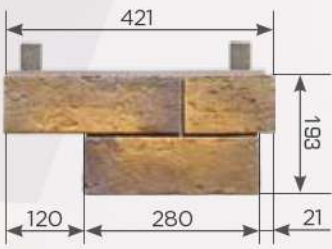
УГОЛ СОСТАВНОЙ ЛЕВЫЙ
