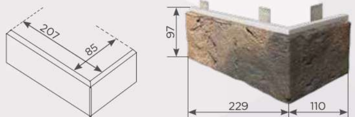
УГОЛ В ПЛОСКОСТИ
