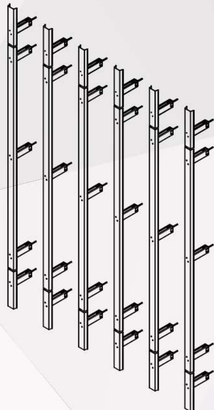
Схема вертикальной подо- блицовочной конструкции
